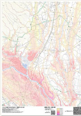
洪水浸水想定区域地図
